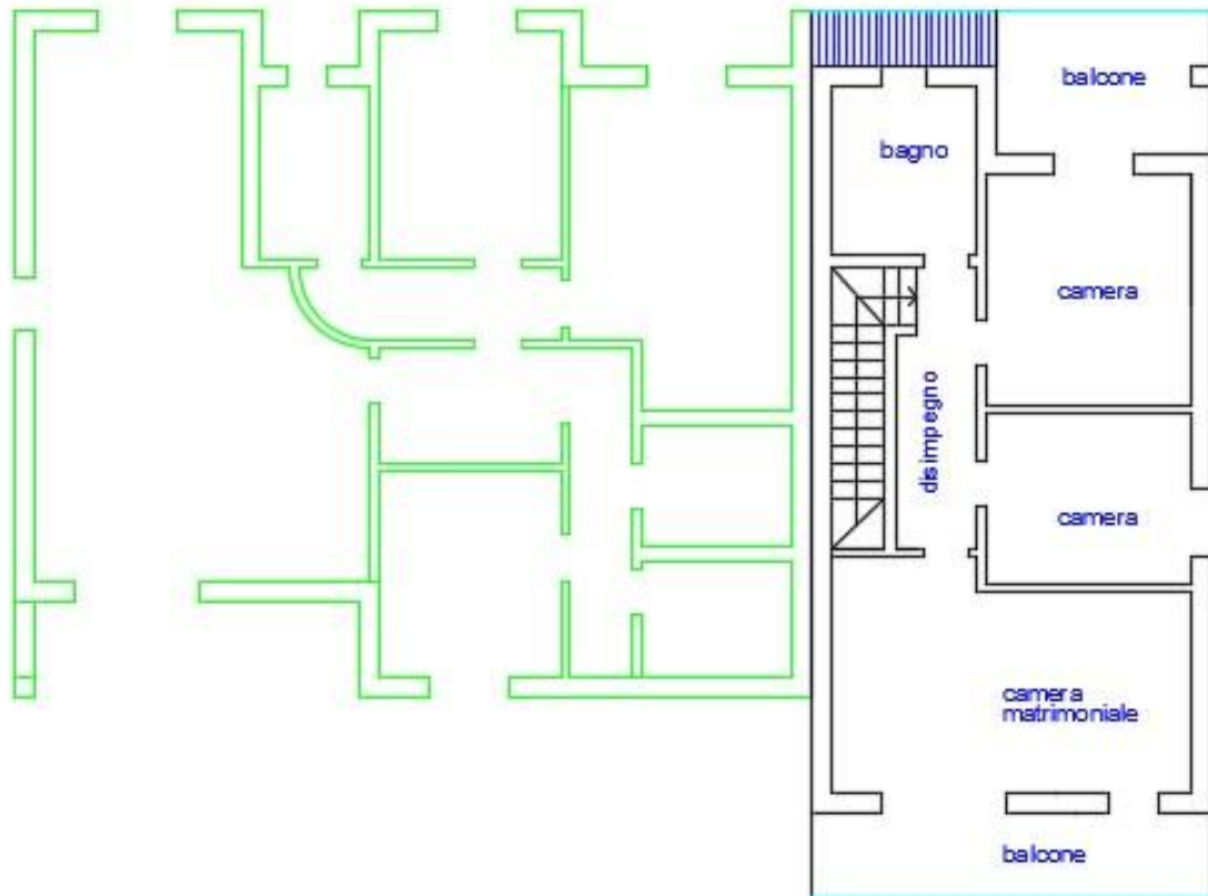
Primo piano
