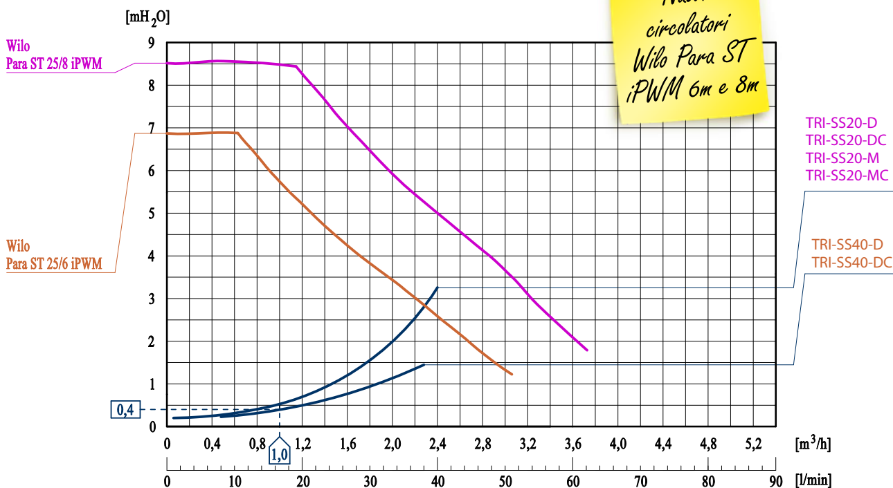
Curve caratteristiche dei moduli e dei circolatori
