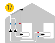
17 Solare con 2 accumuli e 2 pompe
