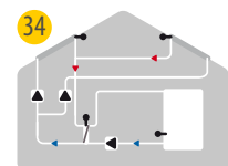
34 2x Solare con accumulatore, scambiatore e 3 pompe
