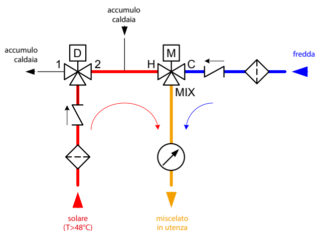
Schema 1: funzionamento con una temperatura dell'accumulo solare superiore a 48°C
