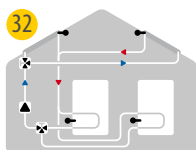
32 Solare con 2 collettori, 2 accumuli e 2 valvole
