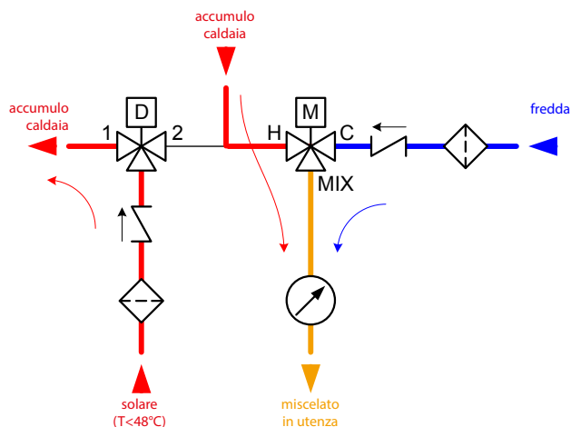
Schema 2: funzionamento con una temperatura dell'accumulo solare inferiore a 48°C
