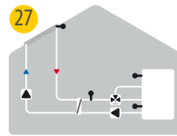
27 Solare con scambiatore e valvola di zona
