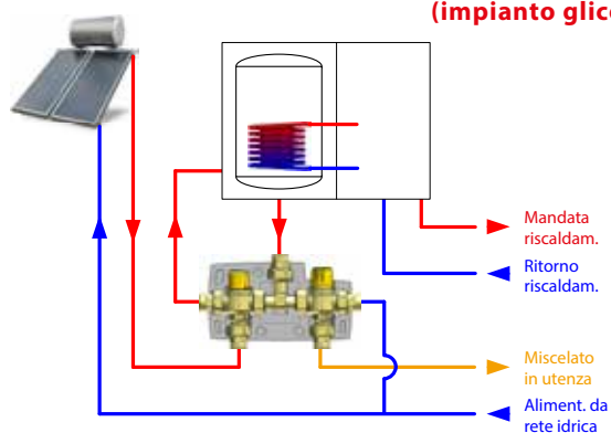
Circolazione naturale (gravità)
