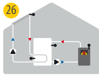
26 Solare con accumulatore e caldaia a legna
