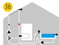
36 Solare con piscina, accumulatore, scambiatore e valvola
