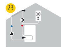
23 Solare con raffreddamento 1 (raffreddamento collettore)
