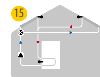
15 Solare con 2 collettori
