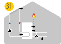
31 Solare con termostato e innalzamento ritorno
