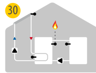
30 Solare con termostato e carico accumulatore
