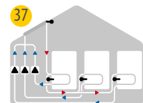
37 Solare con 3 accumuli e 3 pompe
