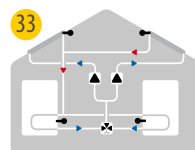
33 Solare con 2 collettori, 2 accumuli e 2 pompe
