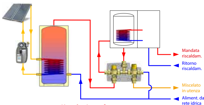
Circolazione forzata (impianto glicole / circuito chiuso)
