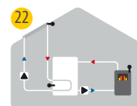
22 Solare con caldaia a legna
