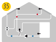
35 2x Solare con accumulatore, scambiatore e valvola
