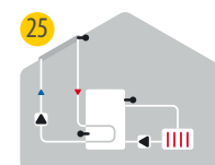
25 Solare con raffreddamento 3 (raffreddamento collettore)
