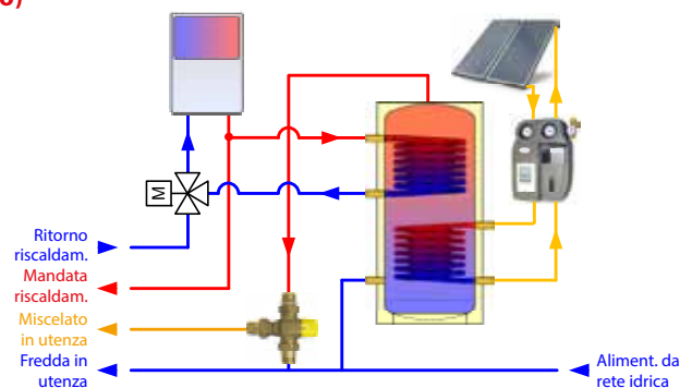
Circolazione forzata (impianto glicole / circuito chiuso) ed integrazione con caldaia
