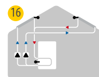
16 Solare con 2 collettori e 2 pompe
