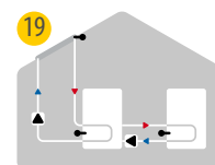
19 Solare con carico accumulo
