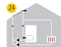
24 Solare con raffreddamento 2 (raffreddamento collettore)
