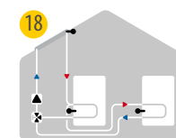
18 Solare con 2 accumuli e valvola
