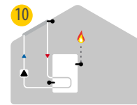
10 Solare con termostato (riscaldamento integrato)
