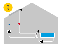
9 Solare con scambiatore calore (sonda sul secondario) e piscina
