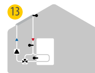
13 Solare con bypass
