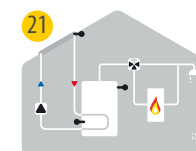
21 Solare con termostato e valvola
