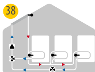
38 Solare con 3 accumuli e 2 valvole
