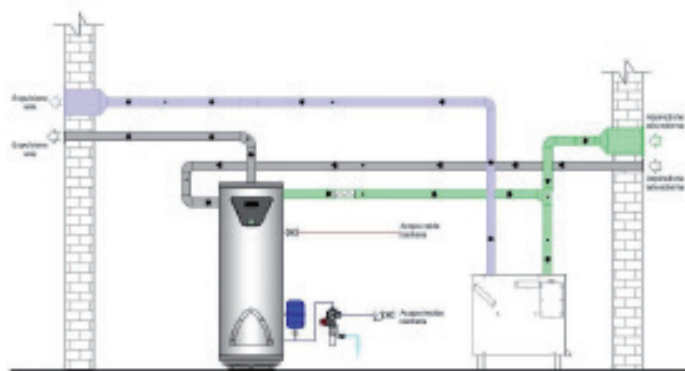
Esempio di collegamento per sinergia con i sistemi MyDATEC
